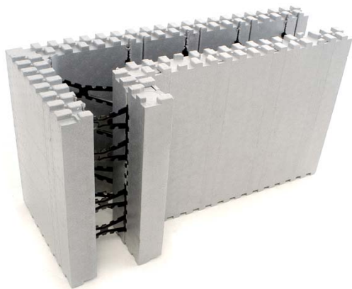
Bild 2 Hörnelement 90
